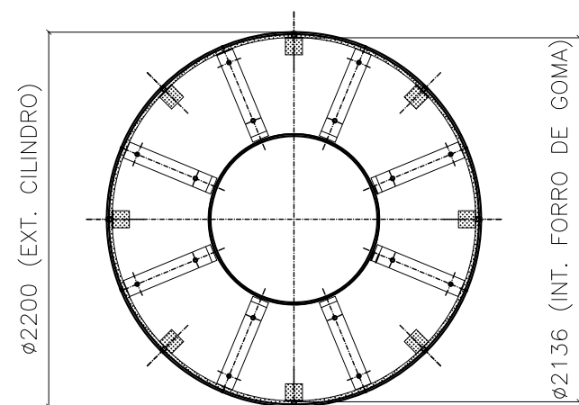
SECCION-DETALLE, ENGOMADO
